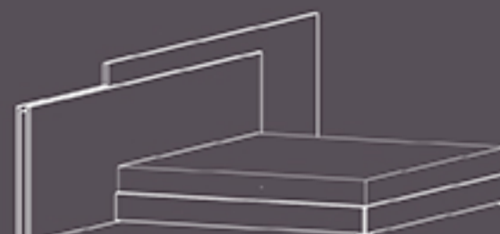
Futura Q.S. bed L 216 W 303 H 108 Futura Lit 154 Futura 160 bed L 216 W 303 H 108 Futura Lit 160 Futura 180 bed L 216 W 331 H 108 Futura Lit 180
